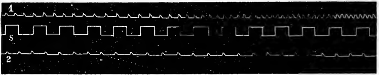
Fig. 89. — Tracés du compte-gouttes : ligne supérieure, liquide versé par le tube de droite; ligne inférieure, liquide versé par le tube de gauche. (Expérience faite sur deux conduits qui versaient de l'eau avec des débits variables.)
